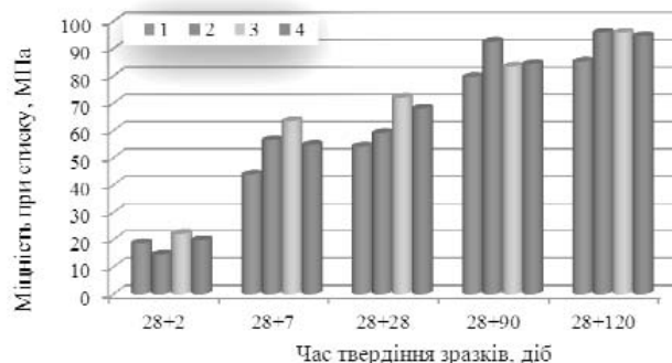
Рис. 2. Кінетика нарощування міцності зразків на основі чистого портландцементу (1) та золацементних композицій, що містять 30 мас.% портландцементу, 6 мас.% крейди і 8 мас.% ангідриту (2) та з добавкою мікрокремнезему у кількості 3 мас.% (3) і 5 мас.% (4) після 28 діб тверднення за температури +3...5 °С та наступного витримування за температури 20±2°С протягом 2, 7, 28, 90 та 120 діб
